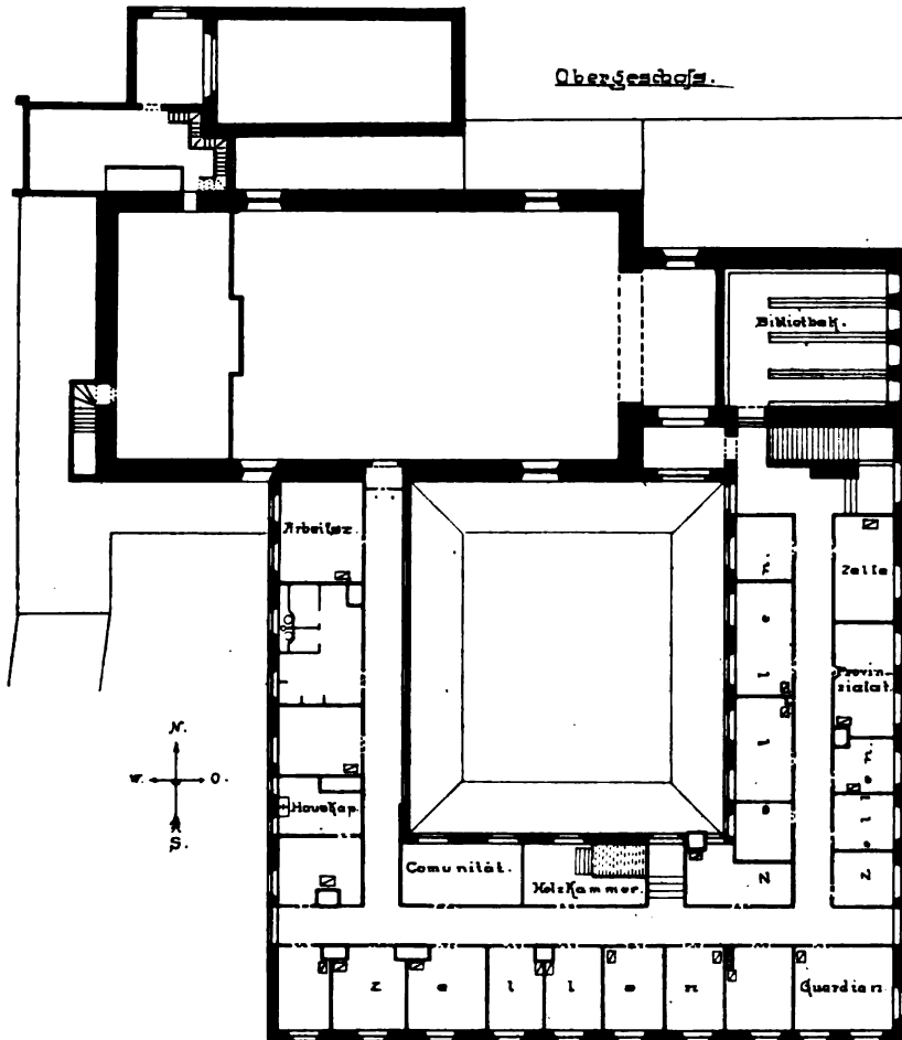
Bild 16. Grundriß des Kapuzinerklosters in Türrheim (zu S. 210).
